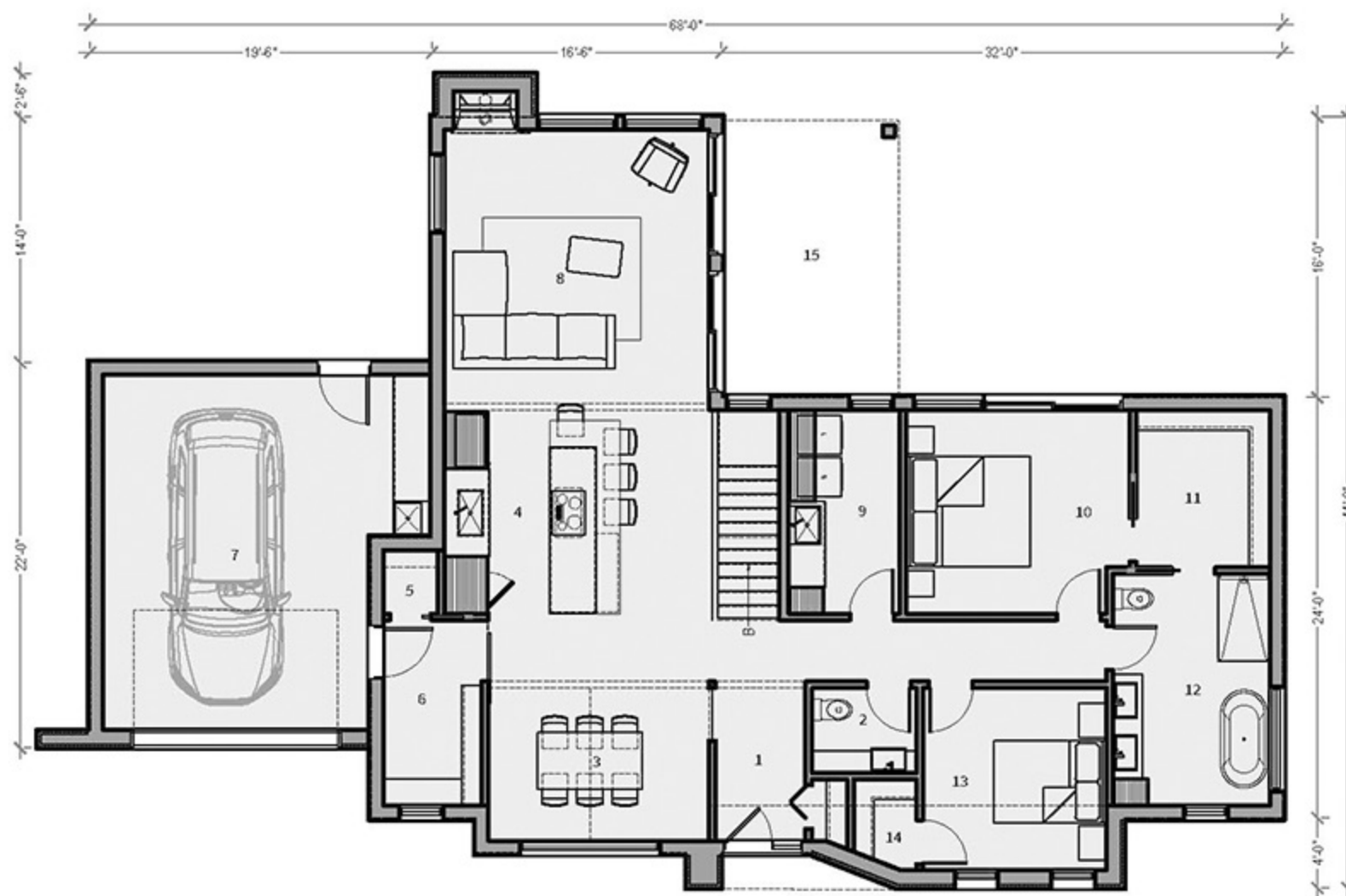
PLAN D'AMÉNAGEMENT - REZ-DE-CHAUSSÉE
